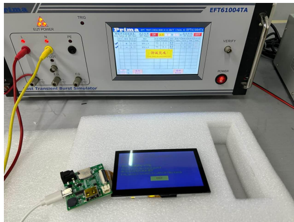
图 6-3 EFT 测试图
