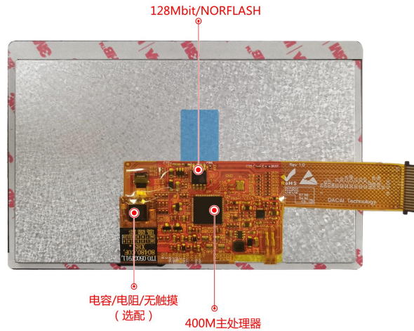
图 1-4 硬件配置图
